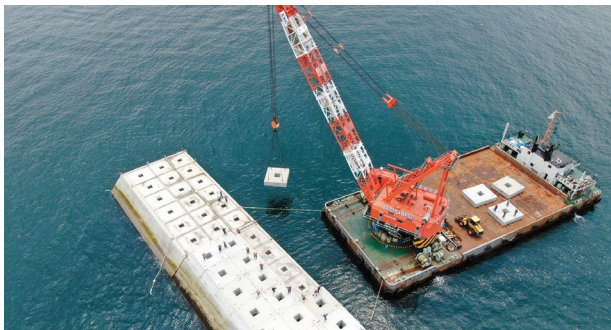
プレキャスト上部工据付状況
