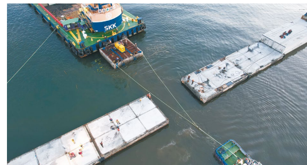
ケーソン据付け作業の様子
