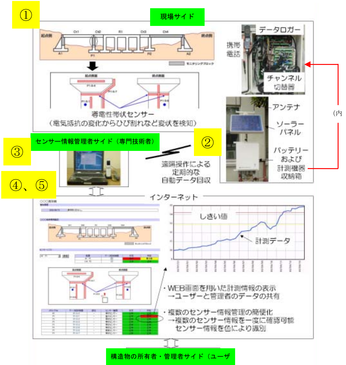
図2：コンクリート構造物の維持管理支援システム「SAMSWING」の概要
